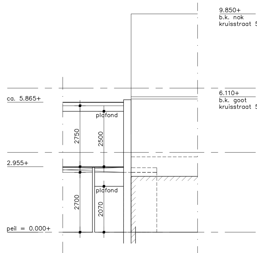
Profiel D-D
