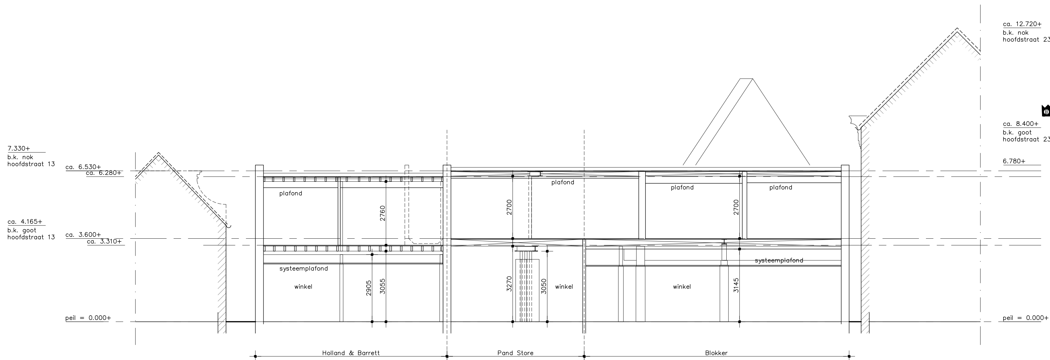
Doorsnede B-B
